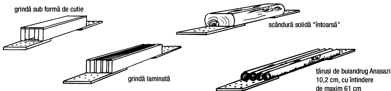
8.1: Tipuri diferite de buiandrug.
