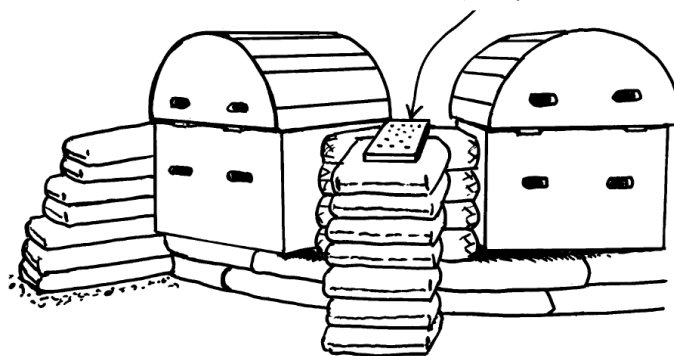
12.14: Încorporarea contraforturilor este o altă metodă pentru a crește masa dintre deschizături și, în același timp, pentru a menține deschizăturile relativ aproape una de cealaltă.
