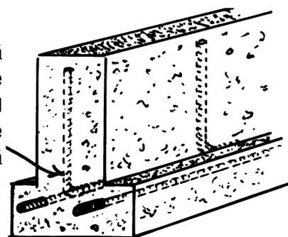
4.2: Vedere a unei secțiuni transversale printr-o fundație obișnuită și prin soclu.
