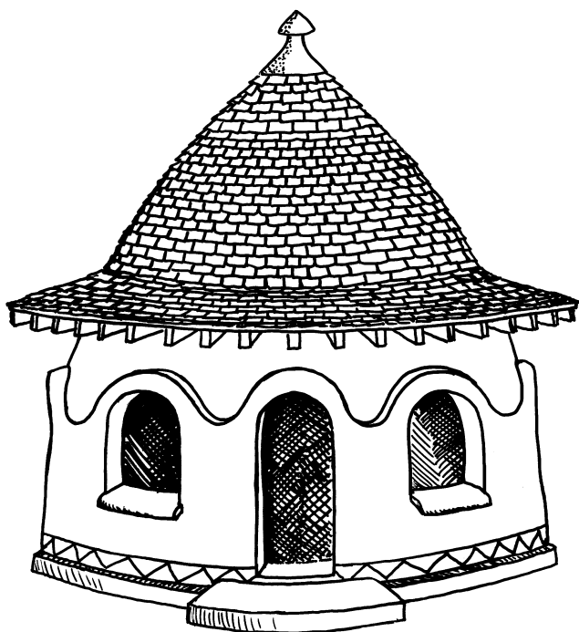
13.8: Șindrițele aplicate direct pe o cupolă din saci cu pământ cu streșini încorporate extinse pentru a proteja pereții.
