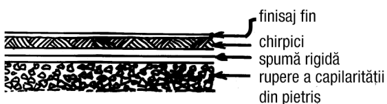
16.2: Trei modalități de izolare a unei podele din chirpici.
