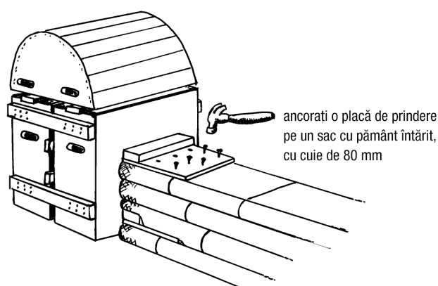
2.29: Benzile de ancorare sunt un punct de sprijin pentru tocurile de uși și anumite tipuri de ferestre.
