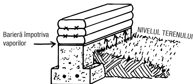
4.9: Membrana impermeabilă la apă previne acțiunea capilarității, împiedicând absorbția apei, prin impunerea unei bariere.
