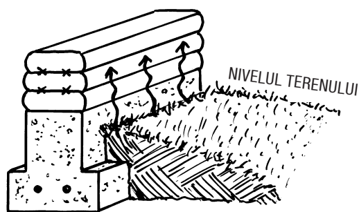
4.8: Acțiunea capilarității: Fără o rupere a capilarității, umezeala din pământ este absorbită de beton și distribuită în părțile mai poroase ale peretelui de pământ de deasupra.
