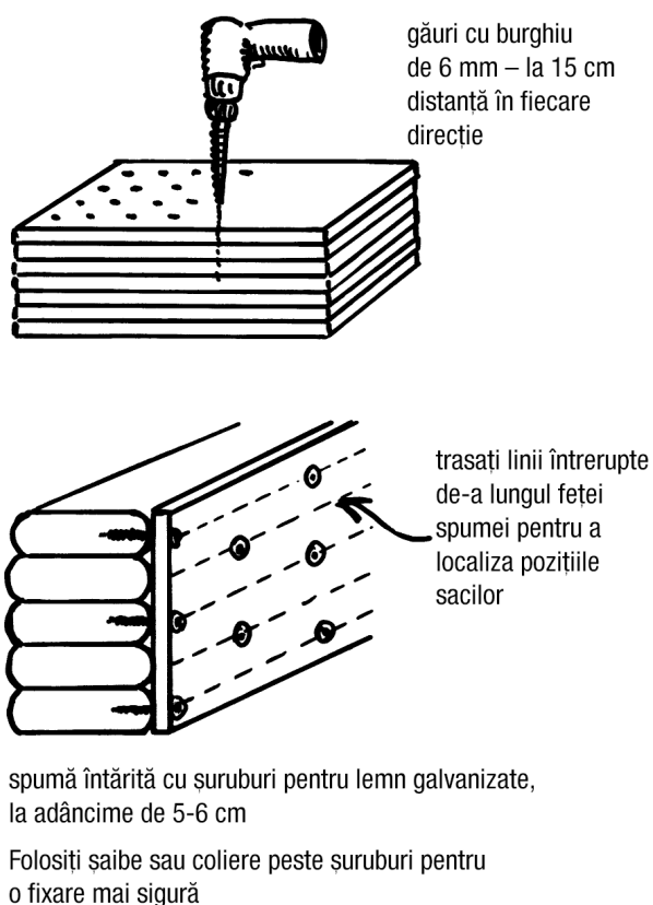
17.7: Pregătirea și atașarea izolației cu spumă rigidă pe un perete din saci de pământ.
