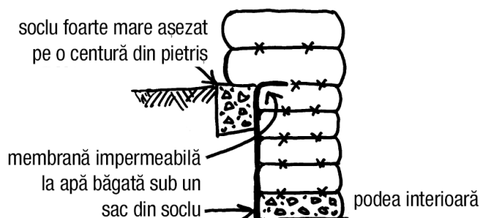
12.10: Detalii ale fundației Honey House.
