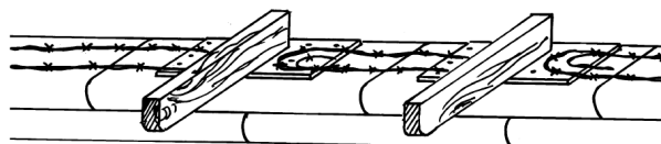
Nivelați peretele cât de mult posibil prin bătătorire, poziționați și prindeți rafturile poliței. Întindeți sârmă ghimpată și următorul rând de saci, bătătoriți, verificați nivelul orizontal din nou, reglați dacă este necesar
