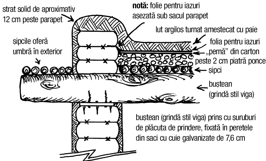
9.31: Izolație exterioră; acoperiș din lut turnat, pentru zonele uscate.
