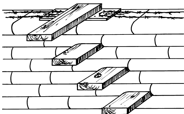
7.13: Amplasați în trepte scânduri pentru scări în timpul construcției, așezate pe plăci de prindere.
