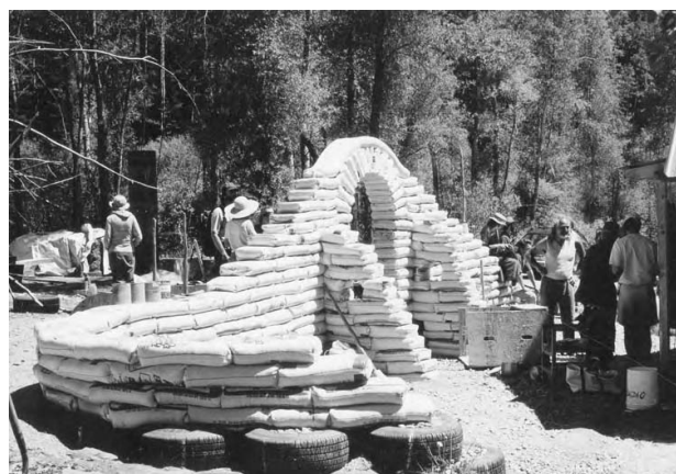
4.13: Fundația/socul menit să susțină un perete din saci cu pământ la workshop-ul din Rico, Colorado, despre clădiri naturale.
