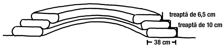
12.1: Test de simulare a curbării făcut pe sol cu tuburi de 38 de centimetri lățime. Exersați tehnica așezării în straturi decalate și testați modul de comportare al pământului vostru.
