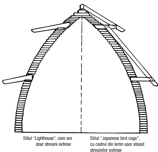
13.9: Cupolă din saci cu pământ cu un cadru de lemn ușor, atasat stresinilor încorporate.
