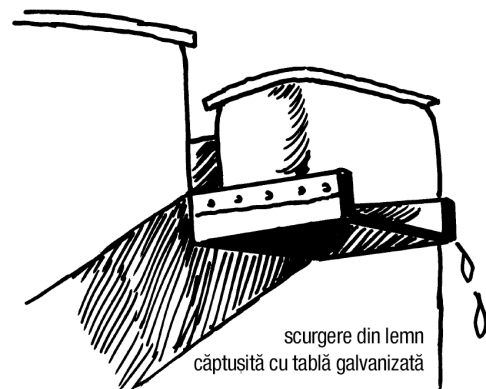
9.15: Stil de scurgere din sud-vest.
