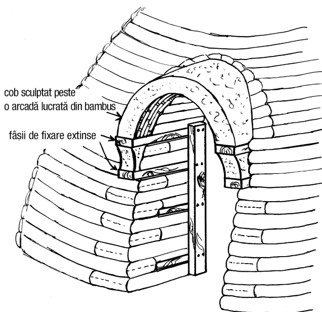
12.15 (jos): Extindeți fâșii extra-lungi de fixare peste profilul zidului și folosiți-le drept poliță pentru a sprijini o fereastră de fronton făcută din cob sculptat, bambus, cărămidă arsă etc. Observație: Consolidarea este extinsă și în interior.
