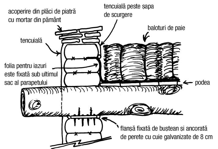
9.29: Detaliu al izolației la un acoperiș boltit cu bușteni stil viga.
