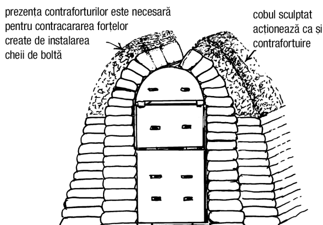
10.13: Fără consolidare suplimentară pe fiecare parte a bolții, cheia de boltă ar forța pereții de sub arcadă.
