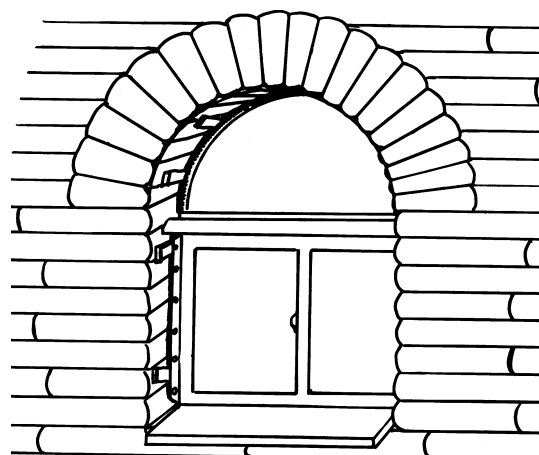
8.5: Fereastră de vinil cu pervaz din lemn fabricat manual și sticlă semicirculară protejată cu garnitură de etanșare din furtun. Ambele ferestre sunt asigurate cu pene până sunt întărite cu tencuiala.
