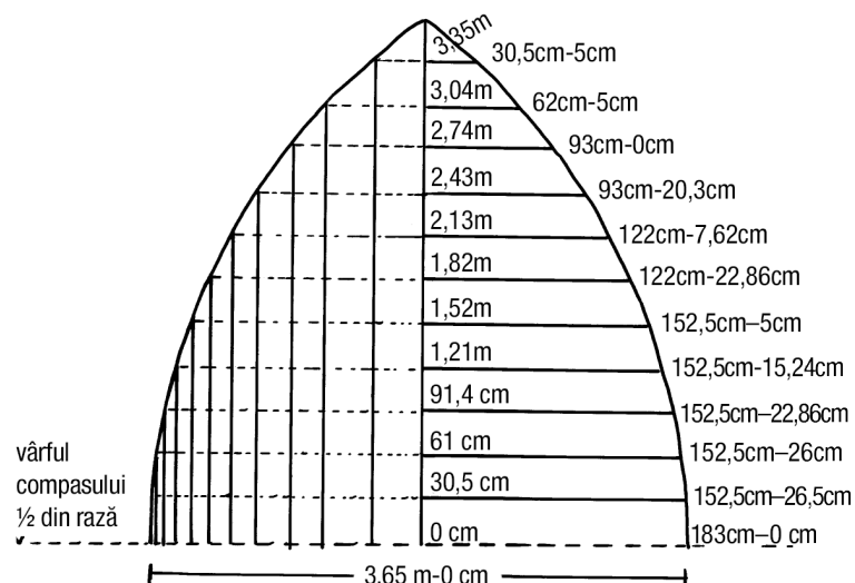
12.17: Această diagramă arată lungimile aproximative la care trebuie ajustat brațul compasului la fiecare 30,5 centimetri înălțime. Puteți desena o diagramă mai mare care să includă măsurători la fiecare doi centimetri sau mai puțin pentru calcule dintr-o privire în timpul construcției.
