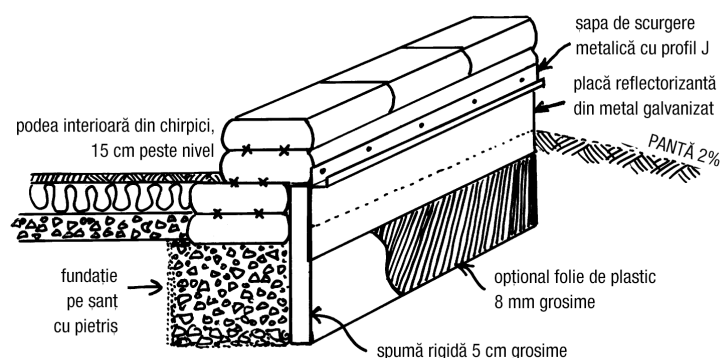
4.14: Fundație de saci cu pământ, izolată.
