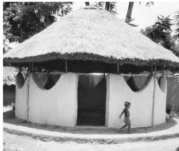
9.32: Cu acoperișul său din paie și cu structura sa din grinzi, stâlpi și umplutură de pământ, casa Baul din Baulkutir, India, se integrează natural în mediul și comunitatea pe care o servește.
