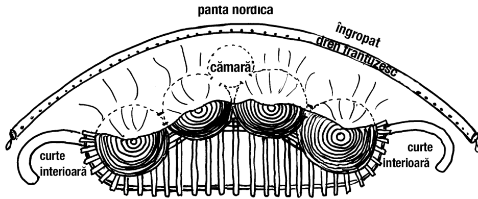
17.4: Patru bordeie interconectate, cu camere în formă de dom îngropate, flancate de pereți de reținere — partea dinspre sud închisă cu o cameră solară atașată pentru climatele reci, sau folosită ca verandă închisă sau marchiză în climatele calde.
