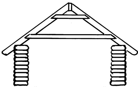
căpriori cu grinzi de coamă și traverse
