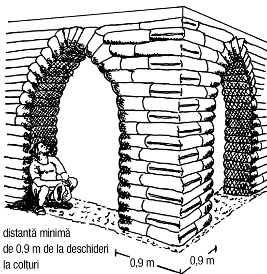
5.10: Alternați saci suprapuși sub formă de zidărie la colțuri pentru un plus de rezistență. Pentru a crește masa în zona amplasării celor două arce în stil egiptean, am construit întregul colț din saci cu lățimea de 50,8 cm și greutatea de 45 kg.
