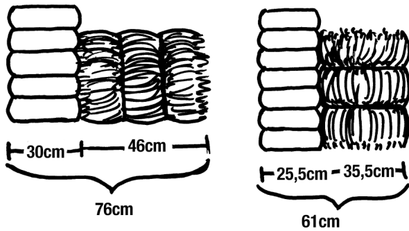
17.9: Configurații alternative pentru saci de pământ și baloți de paie folosiți pentru a obține masă și izolație.
