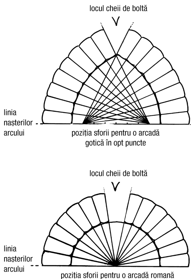
10.7: Exemple de arcadă gotică și romană cu pozițiile sfoarii și locul cheii de boltă.
